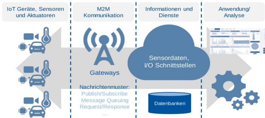
Abbildung 1: Architektur von IoT Systemen (Quelle: Herle et al. 2018)
