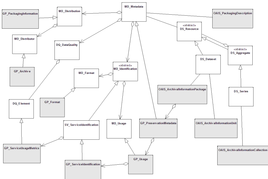
Abbildung 2: Struktur der Klassen für die Archivierung. Weiß: vorhandene Klassen; grau: neue Klassen der ISO 19165-1; MD = Metadata, SV = Services, GP = Preservation.
