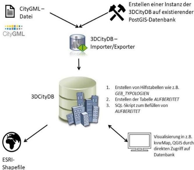
Abbildung 1: Systemarchitektur des Prozesses zur Ableitung der identifizierten Parameter in 3DCityDB. Eigene Darstellung
