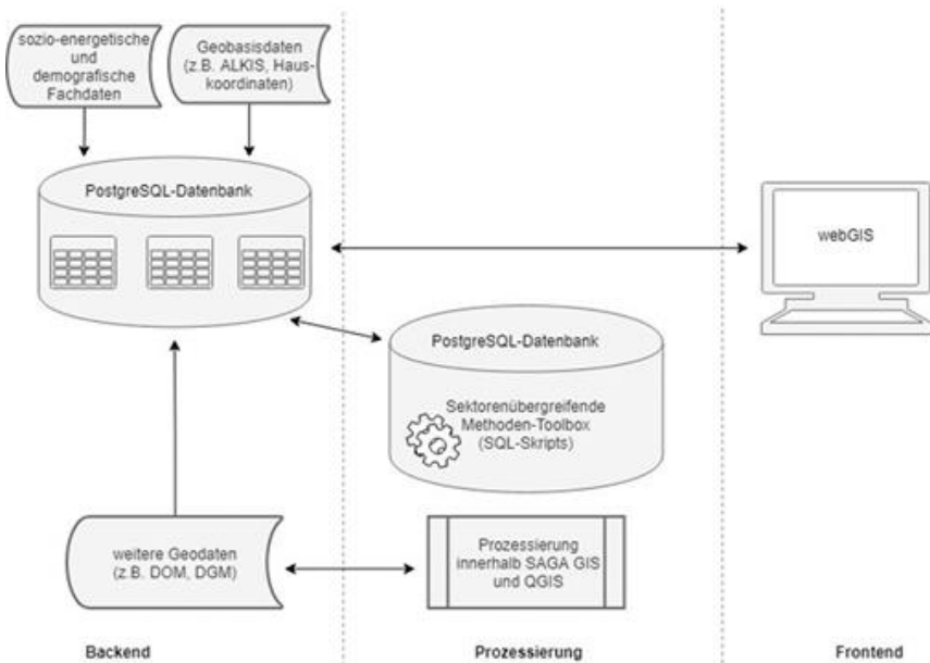
Abbildung 3: Schematische Darstellung der Architektur des GeoEIS
