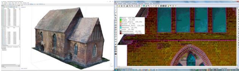
Abbildung 11: Backsteinkirche, Wand-Orthofoto, automatische Steinerkennung
