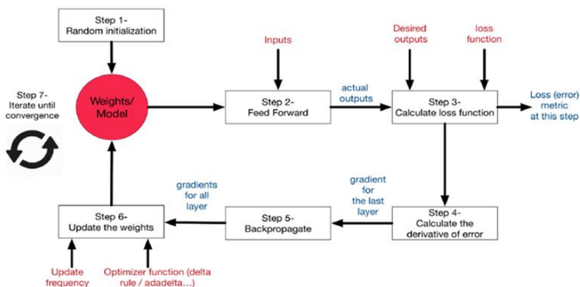
Abbildung 1: Sukzessives Anpassen der Parameter im Neuronalen Netz durch den Prozess der Feed-forward- und Backpropagation (Moawad 2018)
