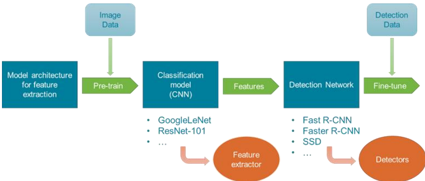
Abbildung 3: Architektur eines Deep Learning Modells zur Objekterkennung (Ellinger 2018)
